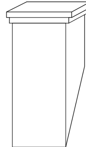
2X Uitkragende rollaag Enkele steenlagen
