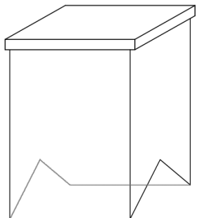
Uitkragende rollaag: Horizontaal, enkele steenlaag
