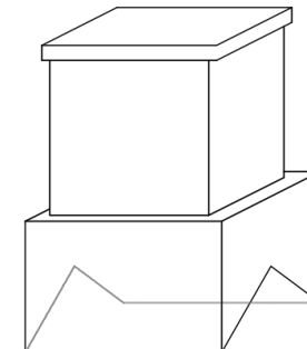
Dubbel uitkragende rollaag: Horizontaal, enkele steenlagen
