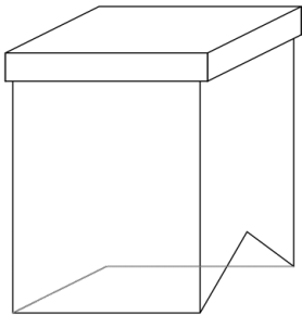
Dubbel uitkragende rollaag: Verticaal + Horizontaal
