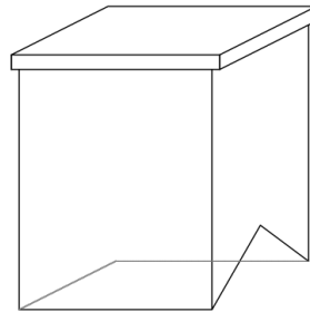
Dubbel uitkragende rollaag: Horizontaal, enkele steenlagen
