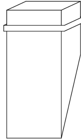
2X Uitkragende rollaag: Enkele + dubbele steenlaag
