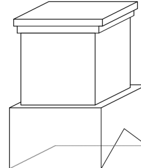
Dubbel uitkragende rollaag: Horizontaal, enkele steenlagen
